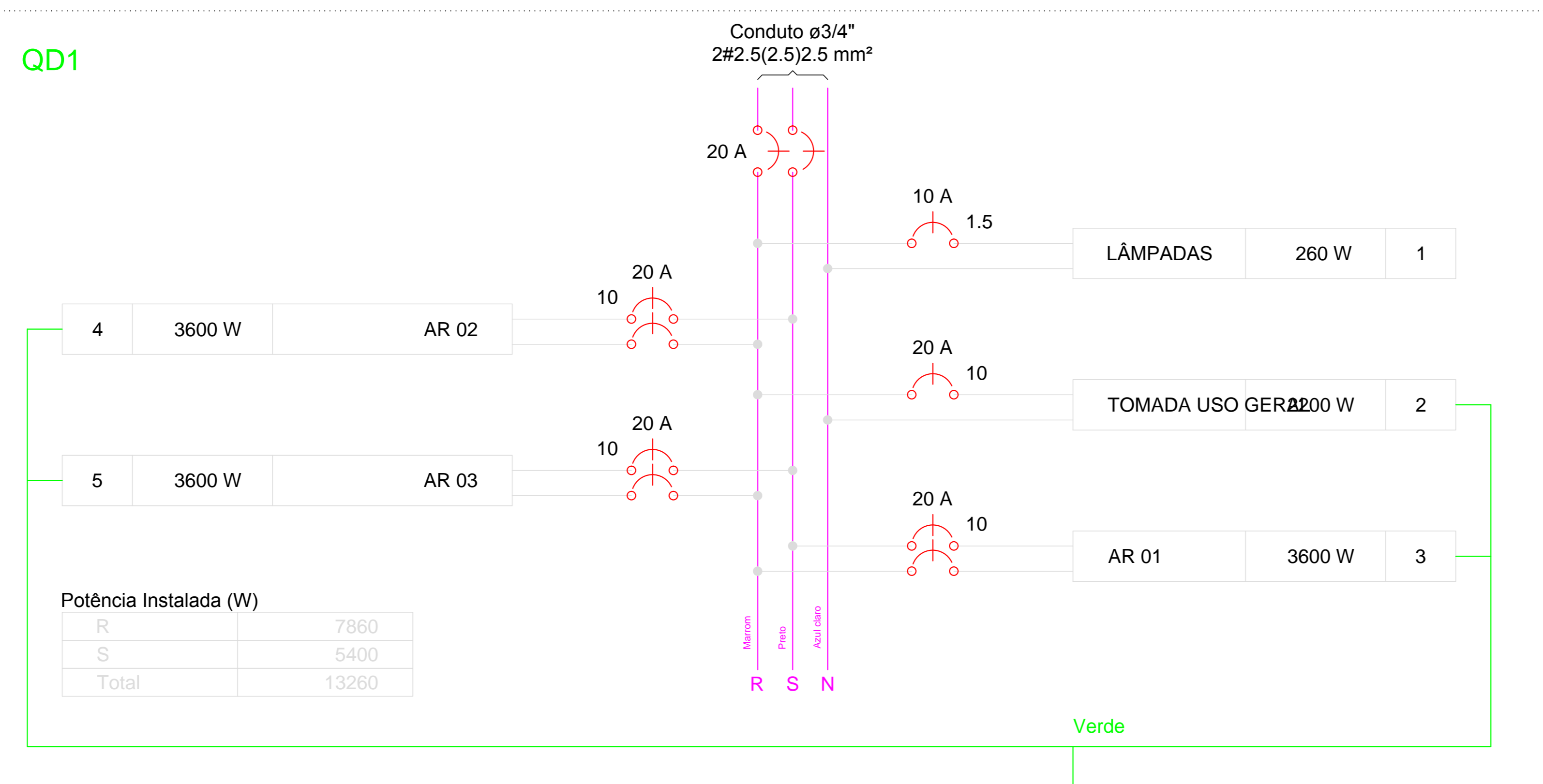
DIAGRAMA MULTIFILAR ESCALA 1: 50
