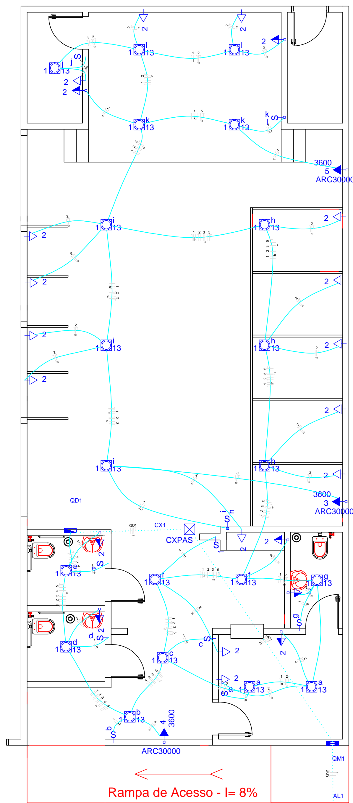
PLANTA PAVIMENTO TÉRREO/ ALTERAÇÃO ESCALA 1: 50
