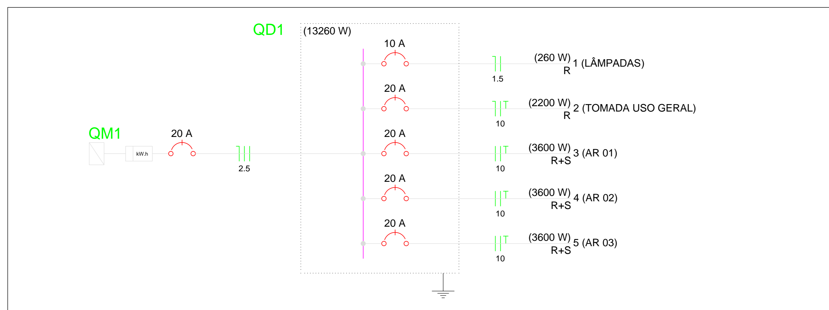
DIAGRAMA UNIFILAR ESCALA 1: 50
