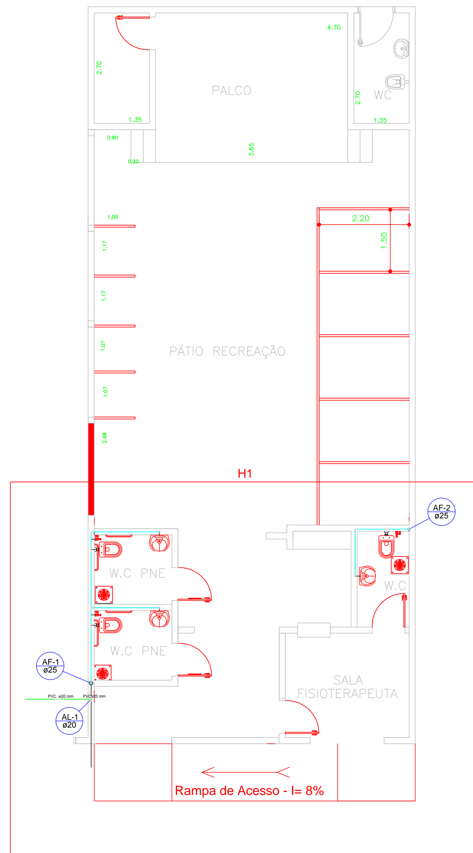
PLANTA PAVIMENTO TÉRREO/ ALTERAÇÃO ESCALA 1:50
