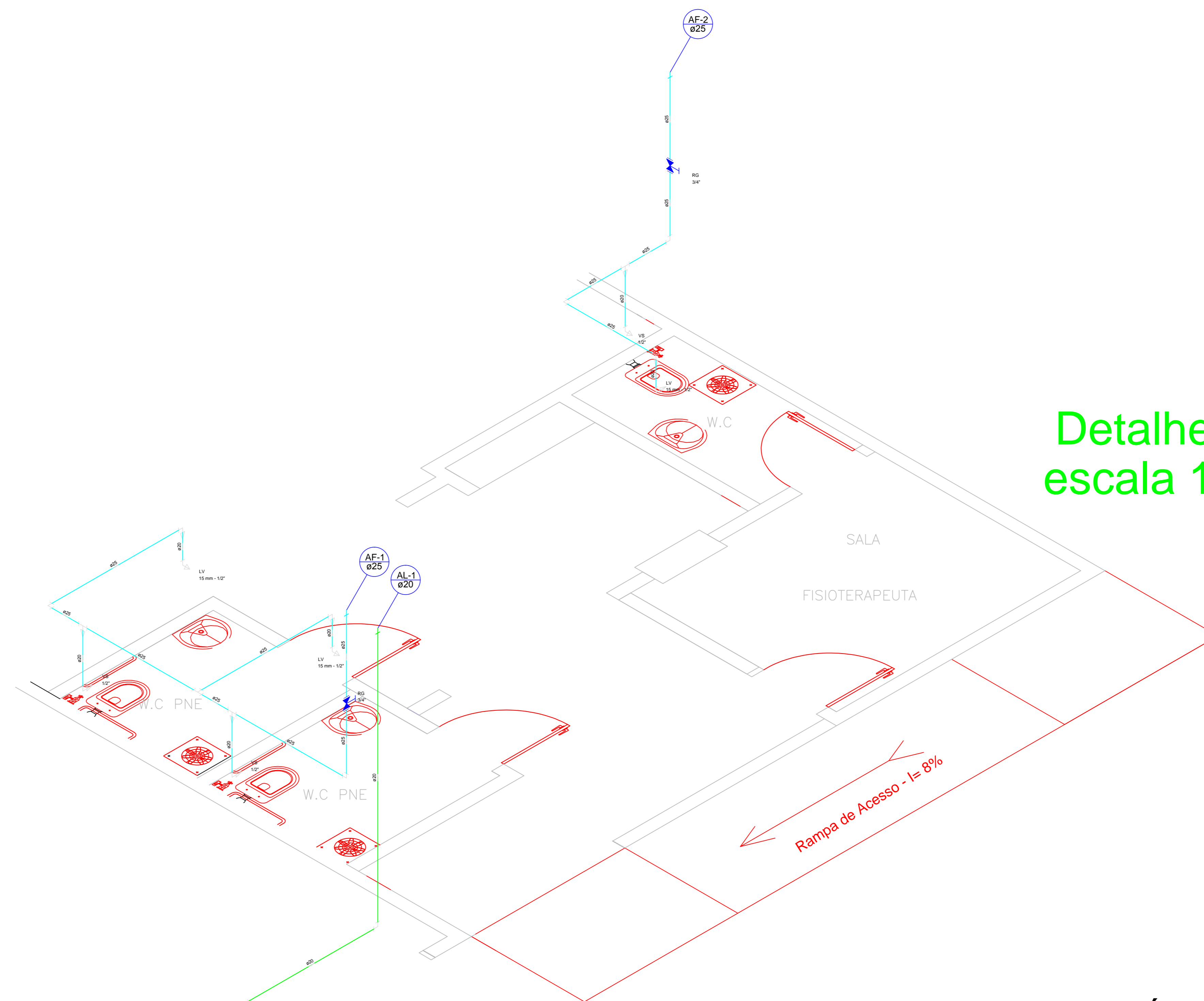
DETALHAMENTO ISOMÉTRICO ÁGUA FRIA ESCALA 1:25
