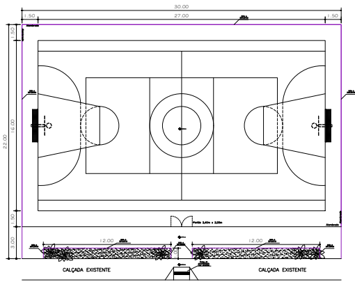
IMPLANTAÇÃO - PRAÇA E QUADRA Esc. 1/100
