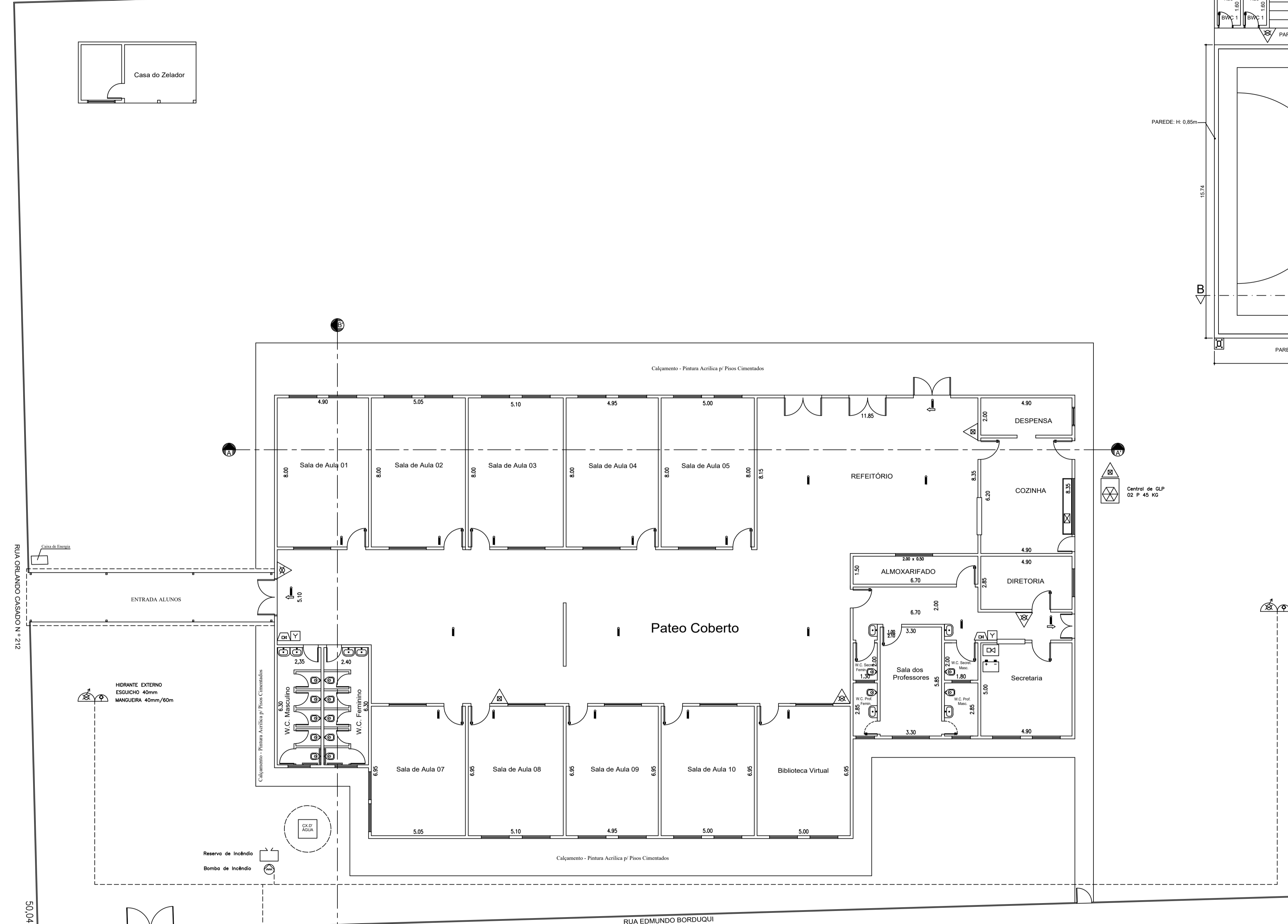
PLANTA ESCALA:1:125
